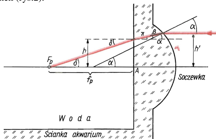
Rys. 2.
